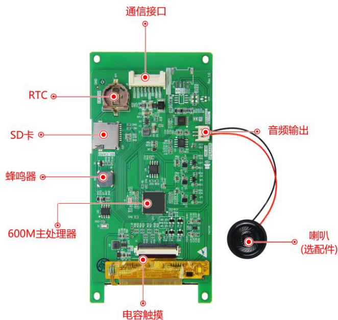
图 1-2 硬件配置图
