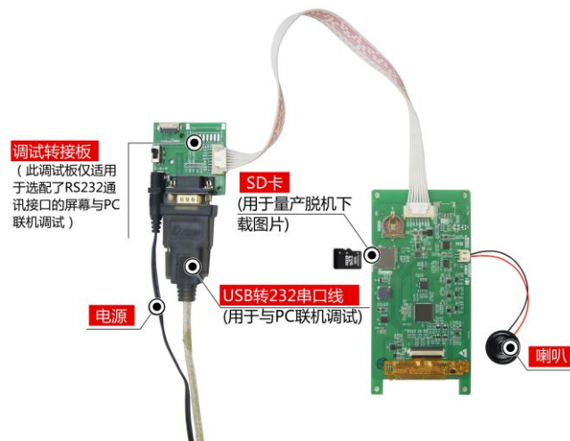
图 1-3 调试工具图
