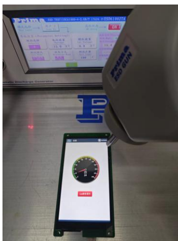
图 4-2 ESD 测试图
